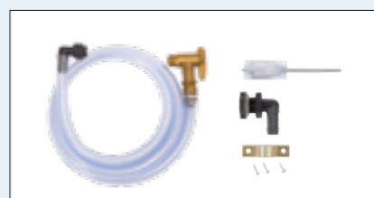
Tuyau jauge universel Indique le niveau de remplissage des réservoirs aériens et permet une utilisation de l'intégralité du volume stocké. Se compose de 2,15 m de tuyau flexible, d'un robinet de soutirage, d'une scie cloche et d'une attache de fixation. S'adapte sur tous les réservoirs aériens. Réf. 220015
